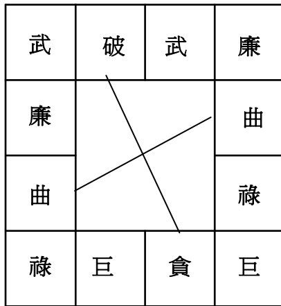
九星圖
