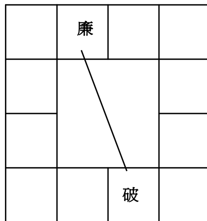
〈地球直徑〉
