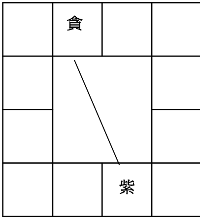
〈北辰〉 〈北極〉
