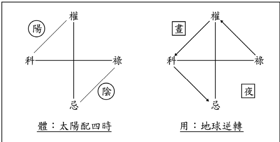
紫微天地圖
