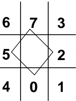
先天易數
