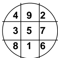
洛書
